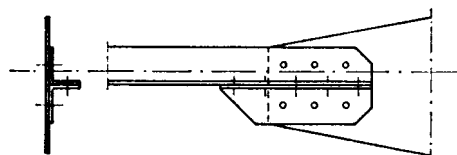
Figure 3.10: Lug angles
